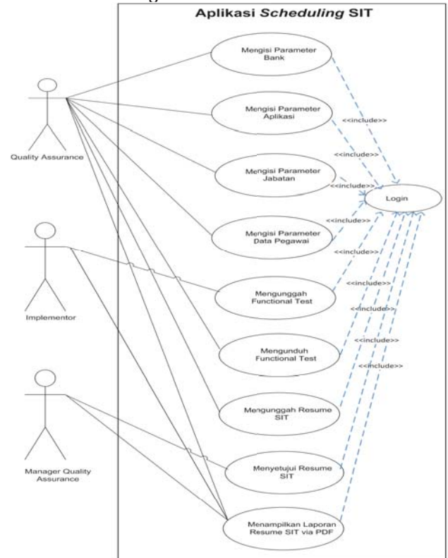
Gambar 3.2 Use Case Sistem Usulan
